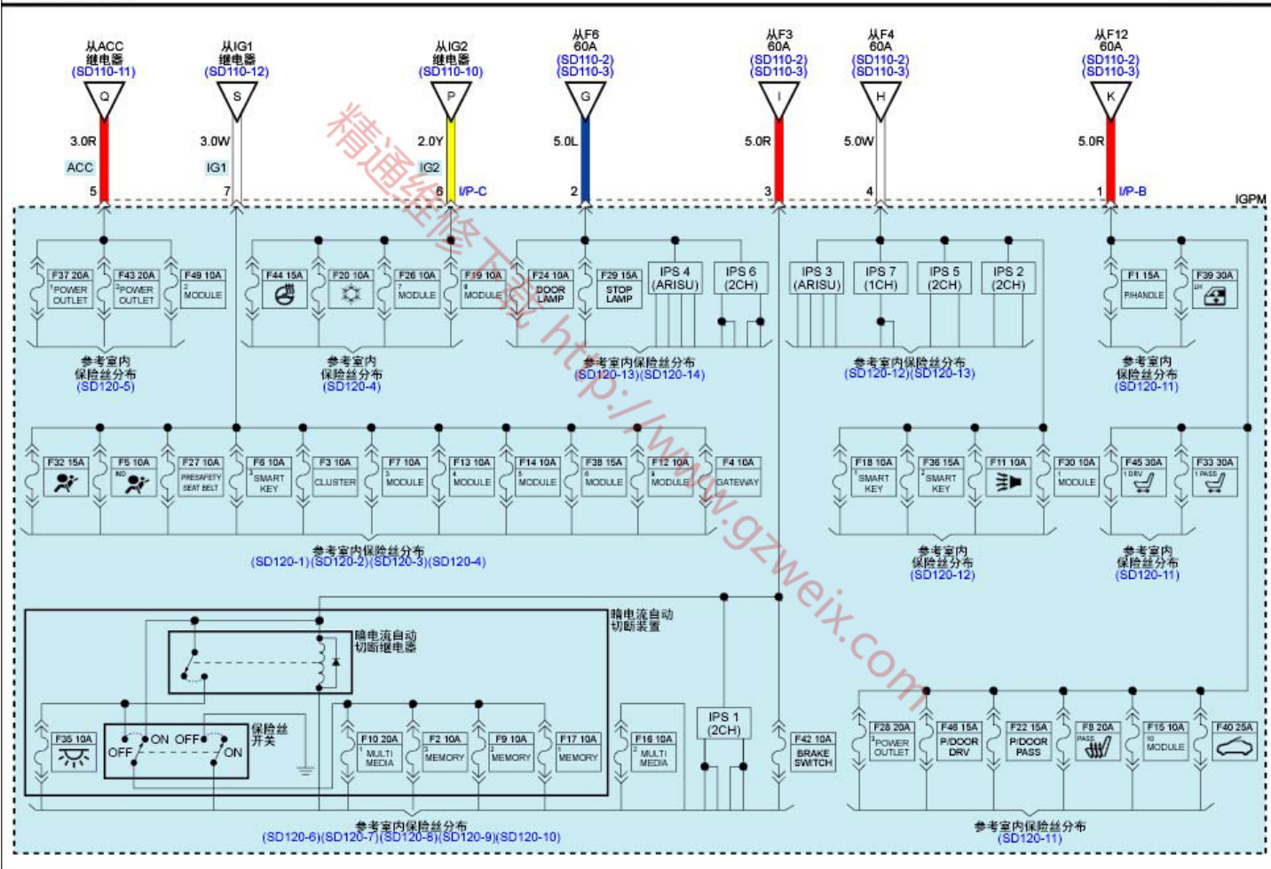
电源分布(13)
